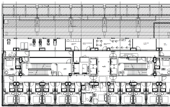
Plan N+1 : Espace hébergement + Zone privée du personnel + Fitness + Laverie Client
