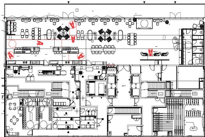
Plan RDC : Zone restauration, Petit déjeuner, Check in + Zone du personnel et Cuisine
